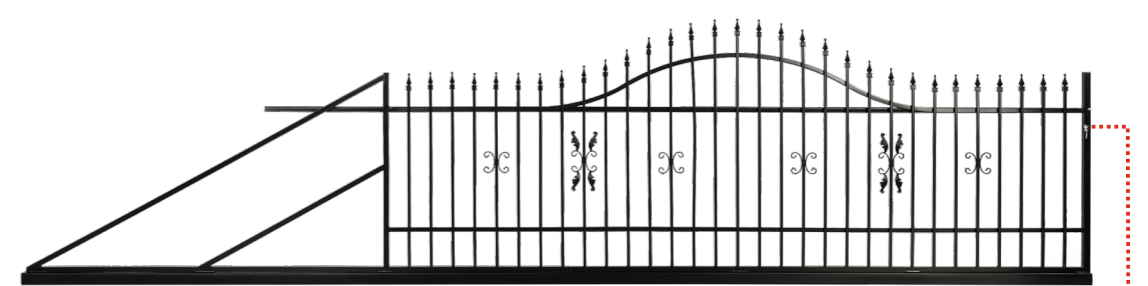
Posuvná brána P/L 4,00 m x 1,20-1,50 m
