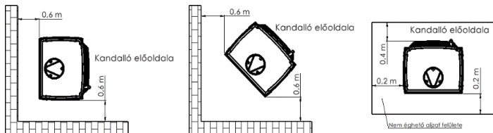
3 sz. Rajz. Biztonságos távolságok a kandallótól
