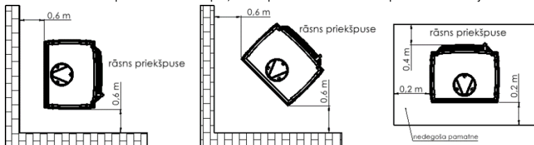
Att. 3 Droši attālumumi no krāsns
