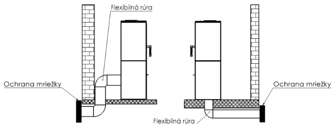
Obr. 2. Schéma pripojenia prívodu vzduchu
