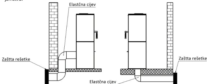
Crtež. 2. Dijagram priklučka za dovod zraka
